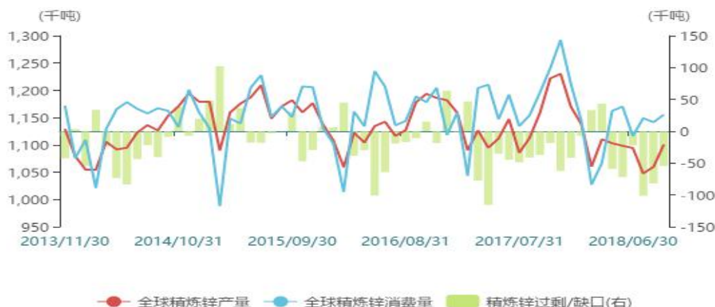
图 4-1：ILZSG 全球精炼锌供需平衡
